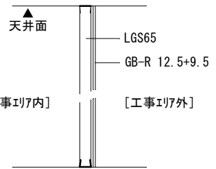
【仮設間仕切り断面図 S=1:30】
