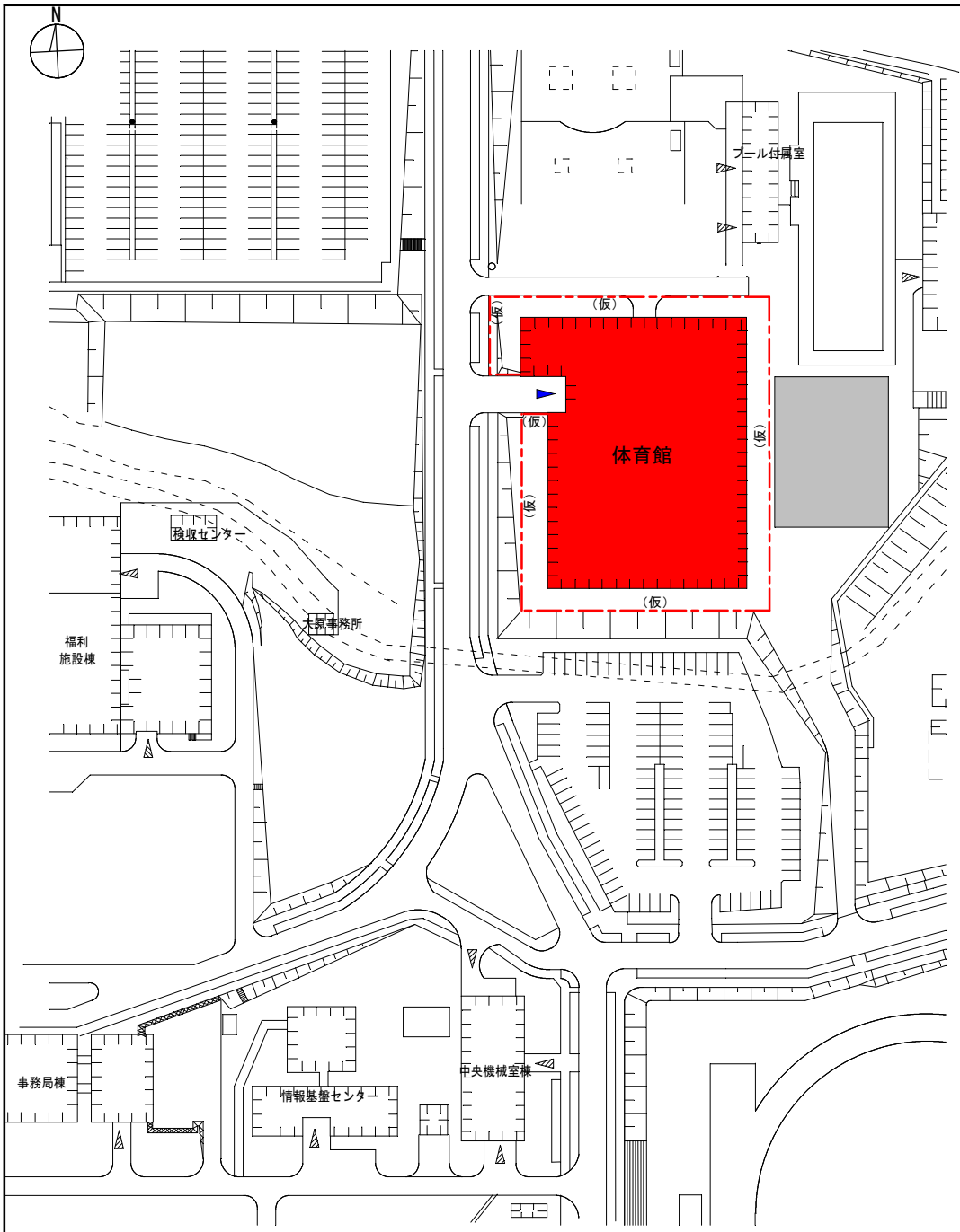
【体育館周辺配置図 S=1:1500】
