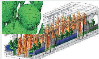
(a) 実環境に基づき構築された数値モデル
