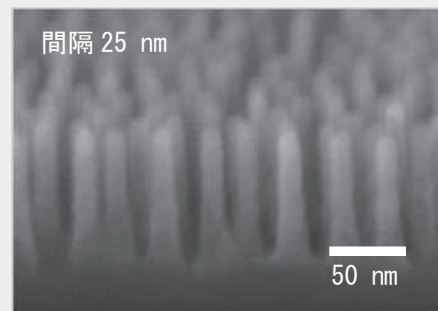
図2:Si 柱状構造の電子顕微鏡像
