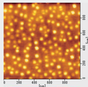
図1:GaAs 量子ドットの電子顕微鏡像
