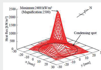
図2 太陽集光部の熱流束分布
