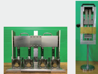
図1 開発中の試作機 (右側: 振動ランマ、左側: 電動ハンマ)
