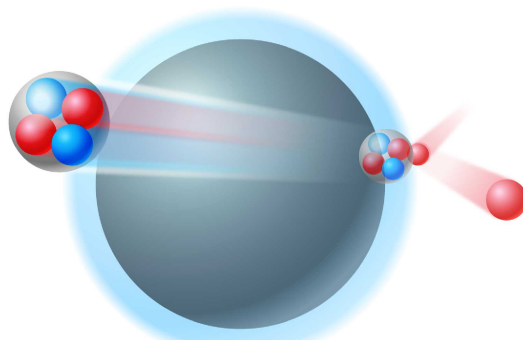
原子核表面のアルファ粒子とノックアウト反応の概念図（赤球が陽子、青球が中性子）
