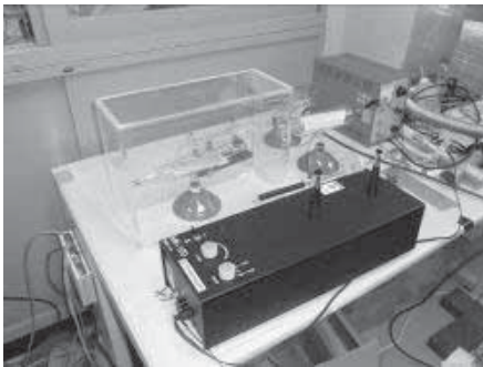
クルックス管および高圧電源
