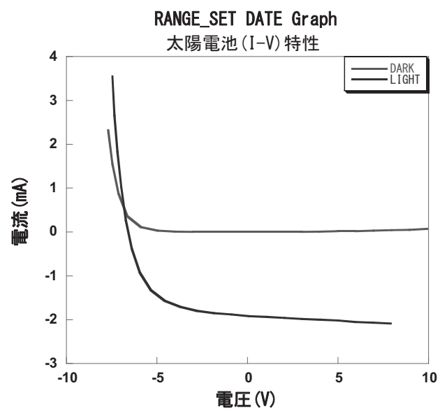
受講生と一緒に TA が作った指導用グラフ (IV 特性)
