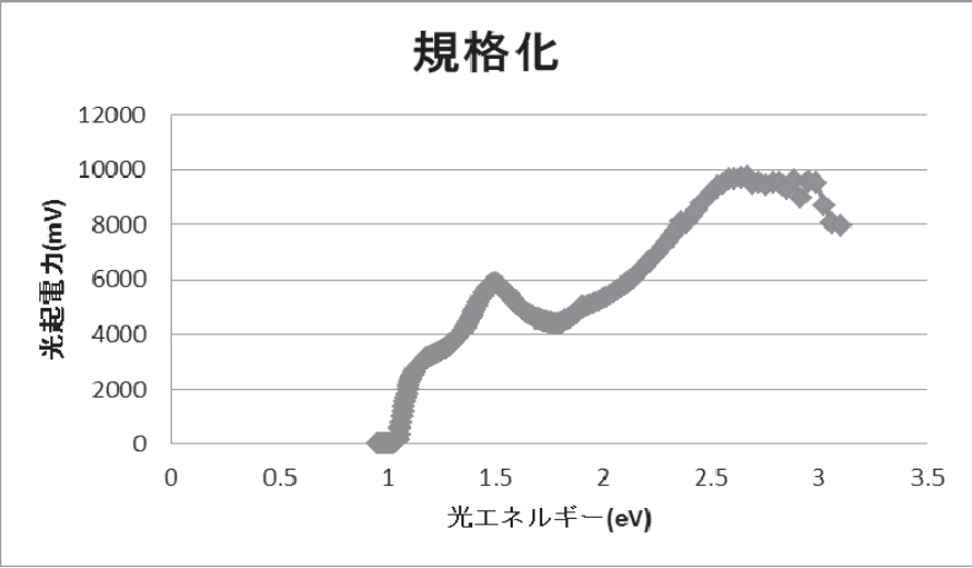
光応答性のスペクトル
