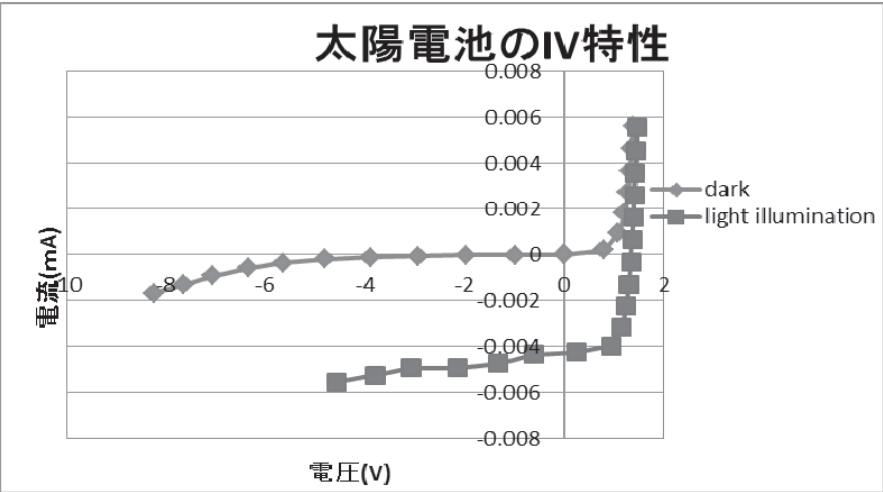
IV 特性の実験結果
