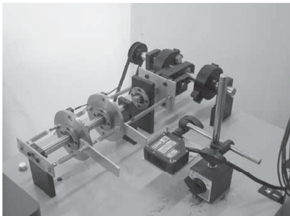
(a) 製作した実験装置
