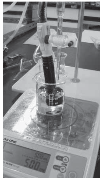
測定器具の設置状況
