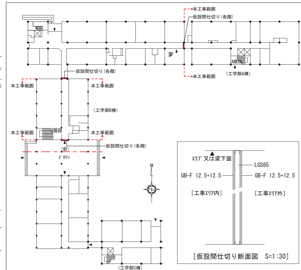
[工学部A棟・B棟内部仮設計画図（標準階）]
