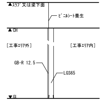
【仮設間仕切り断面図 S-1:30】
