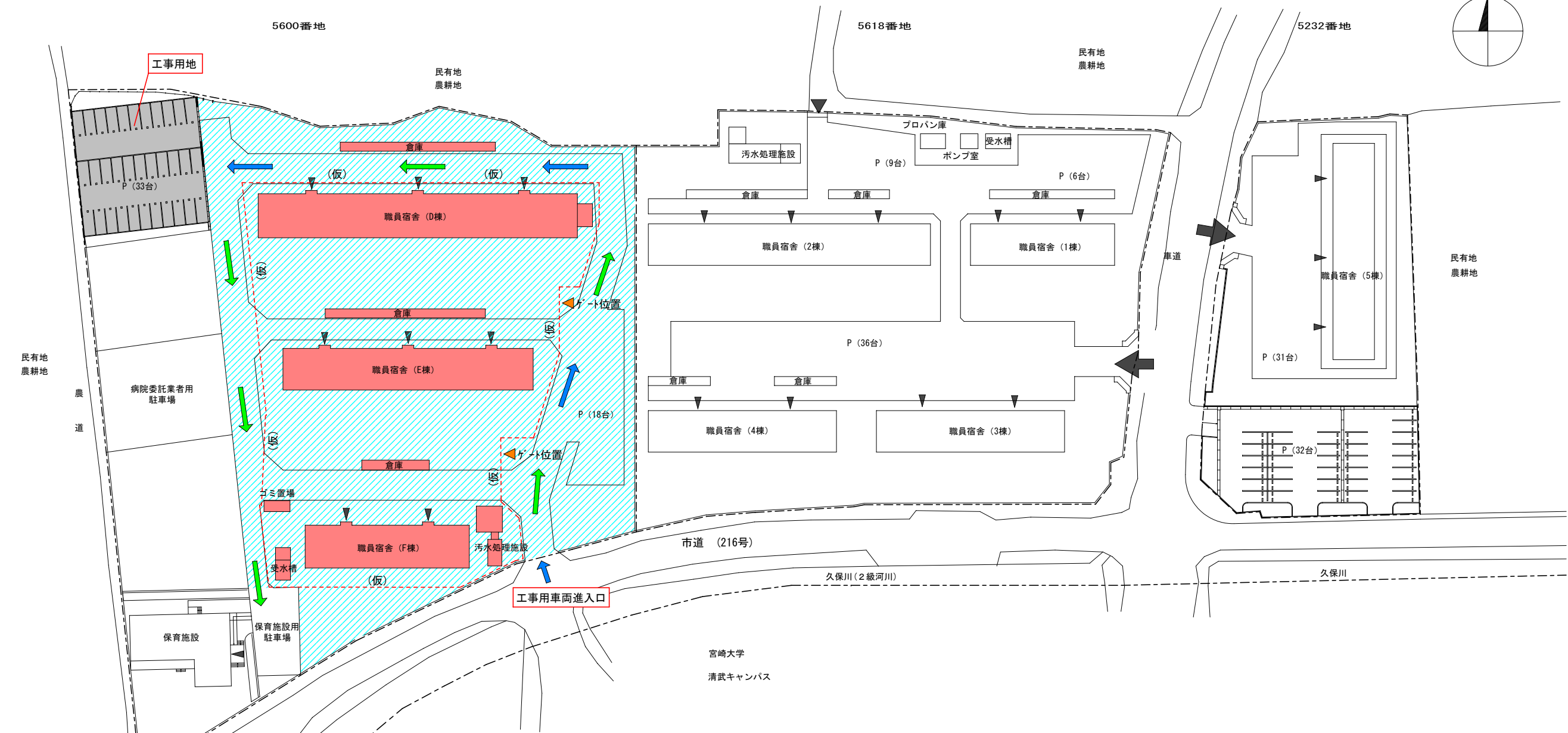
清武 2 団地 配置図 S=1/900
