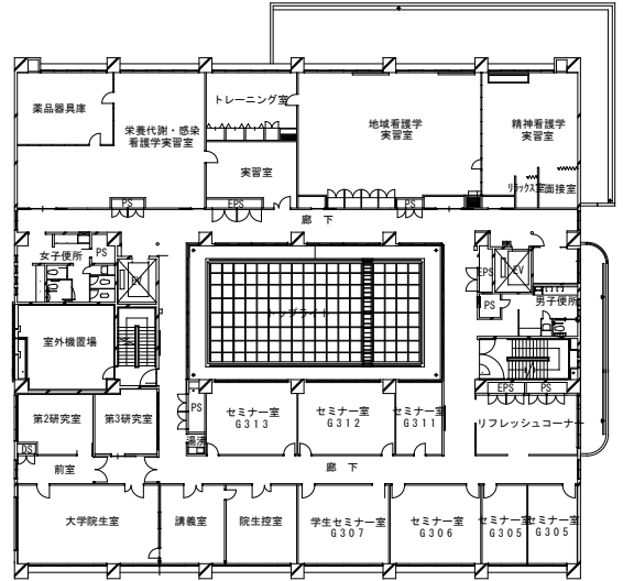
総合教育研究棟 3階平面図
