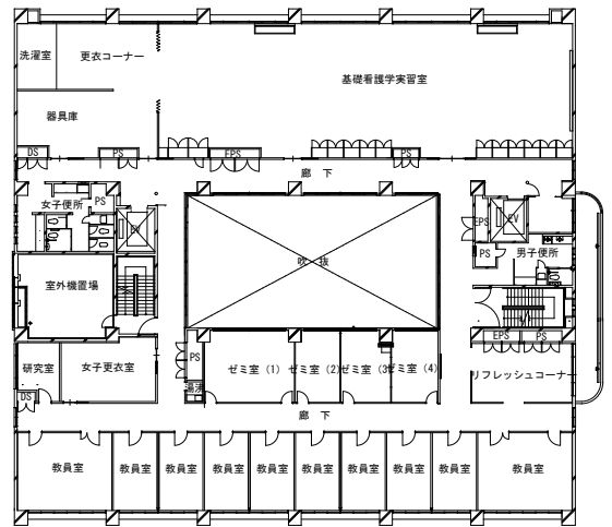
総合教育研究棟 4階平面図
