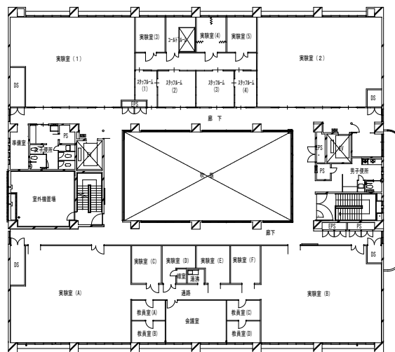
総合教育研究棟 7階平面図
