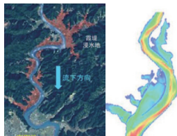
延岡市北川の霞堤位置と その氾濫シミュレーションの例
