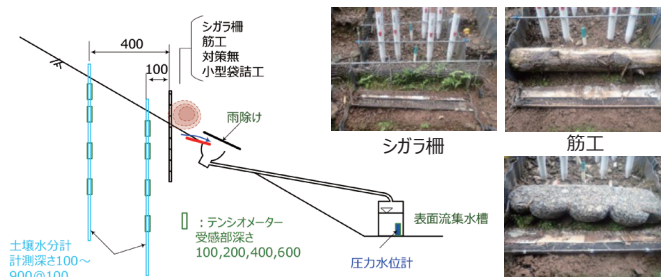
簡便治山工と計測機器設置図
