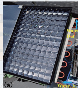
集光型太陽光発電-熱給湯器複合システムの実証実験
