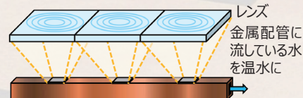
集光型太陽光発電-熱給湯器複合システムの模式図。レンズで集光することで太陽電池のコストを削減
