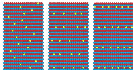
原子層エピタキシー法で意図的に原子分布を変化させた半導体結晶の模式図
