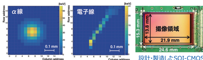
開発した半導体イメージセンサで観測したα線(左)と電子線(右)
