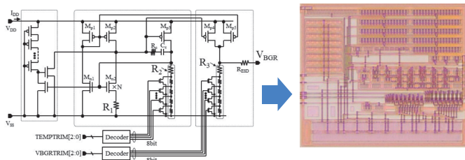
アナログ集積回路の設計(超低電圧参照電圧源回路の回路図とそのチップ写真)
