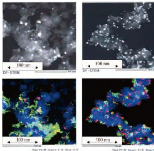
Pt-TiO x /C触媒の透過型電子顕微鏡(TEM)写真、平均粒径6nm以下、白金とチタンの存在ヶ所一致率 90% 以上
