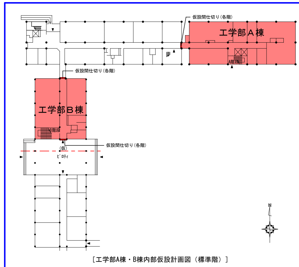
【工事範囲平面図】
